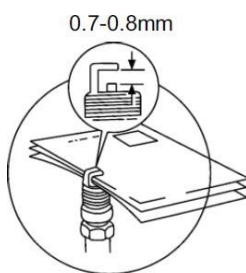
4. Se măsoară distanța dintre electrozi.
